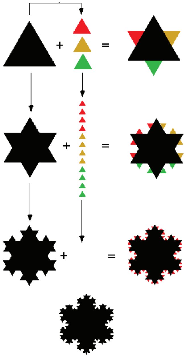
Slika 2: Nastanek Kochove snežinke. (Vir slik: http://mathforum.org/mathimages/index.php/Koch_Snowflake (10. 2. 2013))
